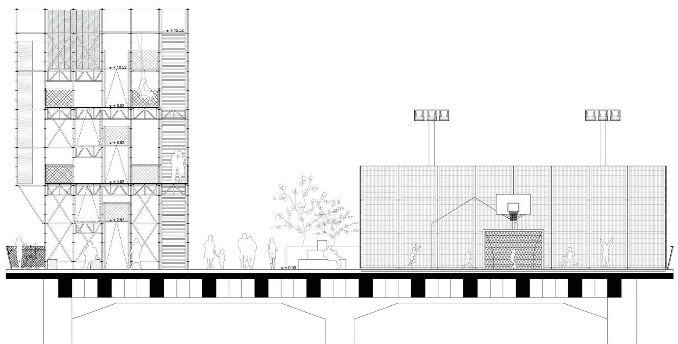
SEZIONE TRASVERSALE scala 1:100
