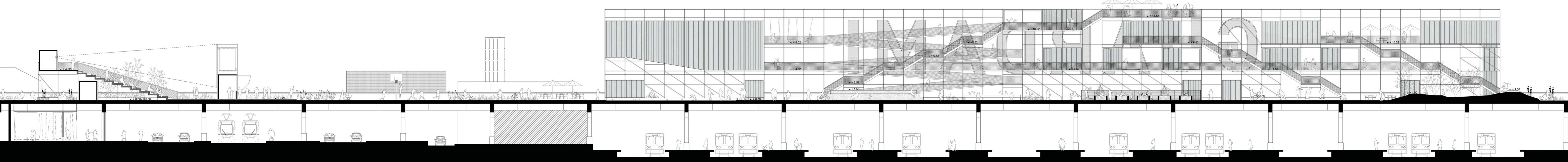
SEZIONE LONGITUDINALE scala 1:200
